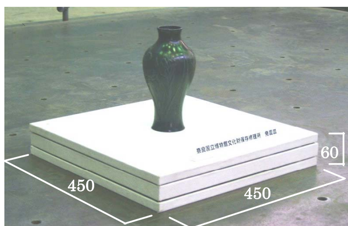
免震皿の例
